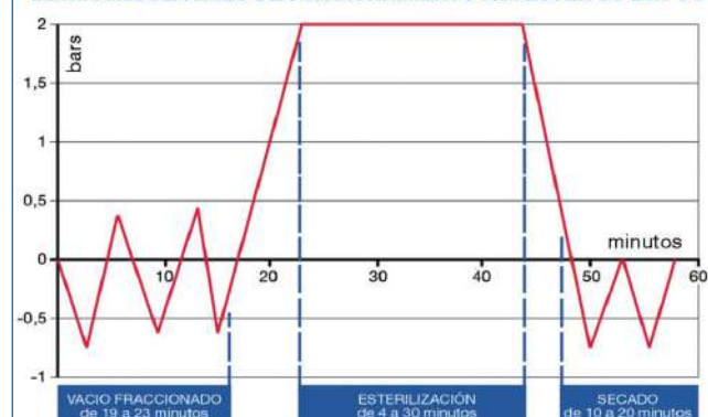
DIAGRAMA DE FASES DE FUNCIONAMIENTO AUTESTER ST DRY PV
