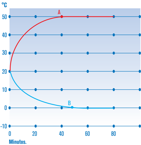
Gráfico de temperatura-tiempo. A. Set a 50 °C: 40'. B. Set a 0 °C: 48'.
